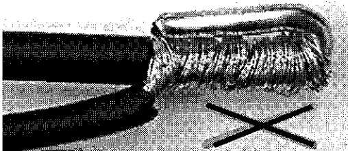
手より結線のイメージ (悪い例)
